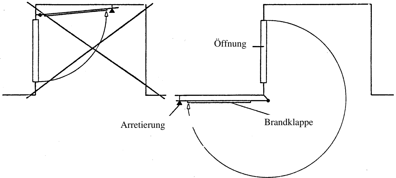
Anordnung einer Brandklappe unterhalb eines Decks
