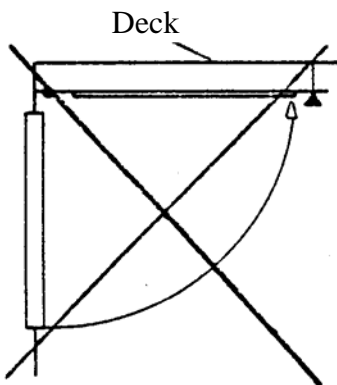
Seitenansicht auf eine Brandklappe - Anordnung der Arretierung am Deck
