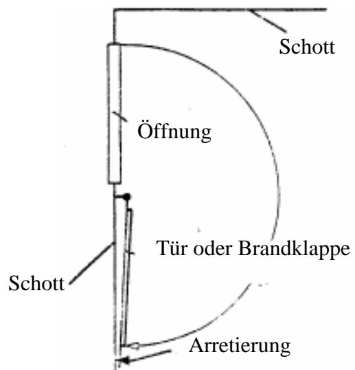
Draufsicht auf eine Tür, die zum freien Deck aufschlägt, bzw. auf eine Brandklappe
