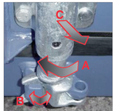
Abbildung 5.28: Betätigung der Türnocken
