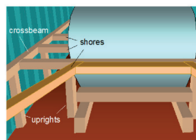
Abbildung 7.5: Aussteifung mit Pfosten und Querträgern
