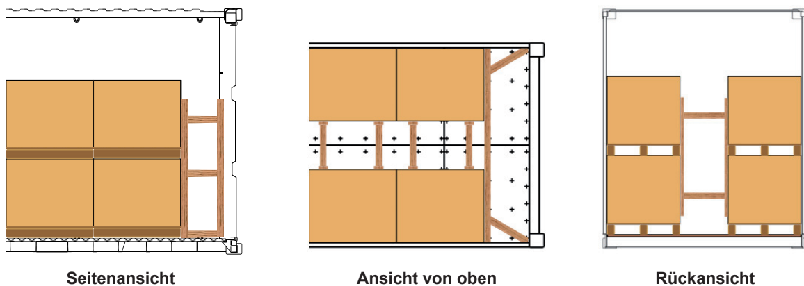
Abbildung 7.32: Dichte Stauung in einer CTU mit soliden Wandungen
